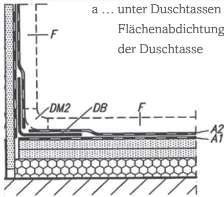
Abb. 11 - Die Eckausbildung und Abdichtung im Spritzwasserbereich. Die Abdichtung „F“ muss hinter den Fliesen fortgeführt werden. [7.12]
