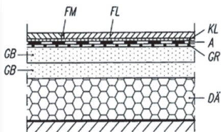
Abb. 13 - Fußbodenaufbau und Abdichtung in der Fläche [7.12]
