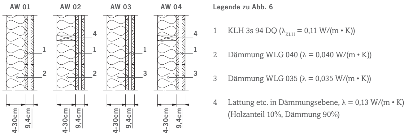
Abb. 6 - Gedämmte KLH- Außenwand (KLH 3s 94 DQ) in vier verschiedenen Varianten
